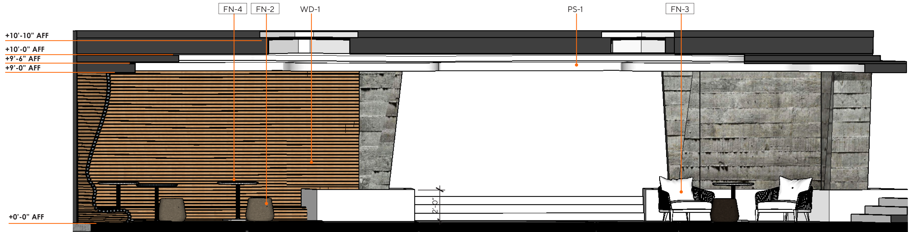
SECTION B1 SCALE: 1/4"=1'-0"
