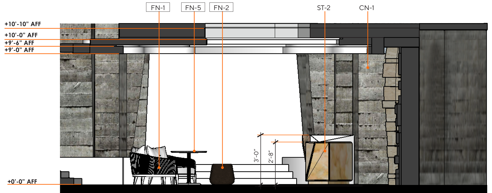
SECTION B2 SCALE: 1/4"=1'-0"
