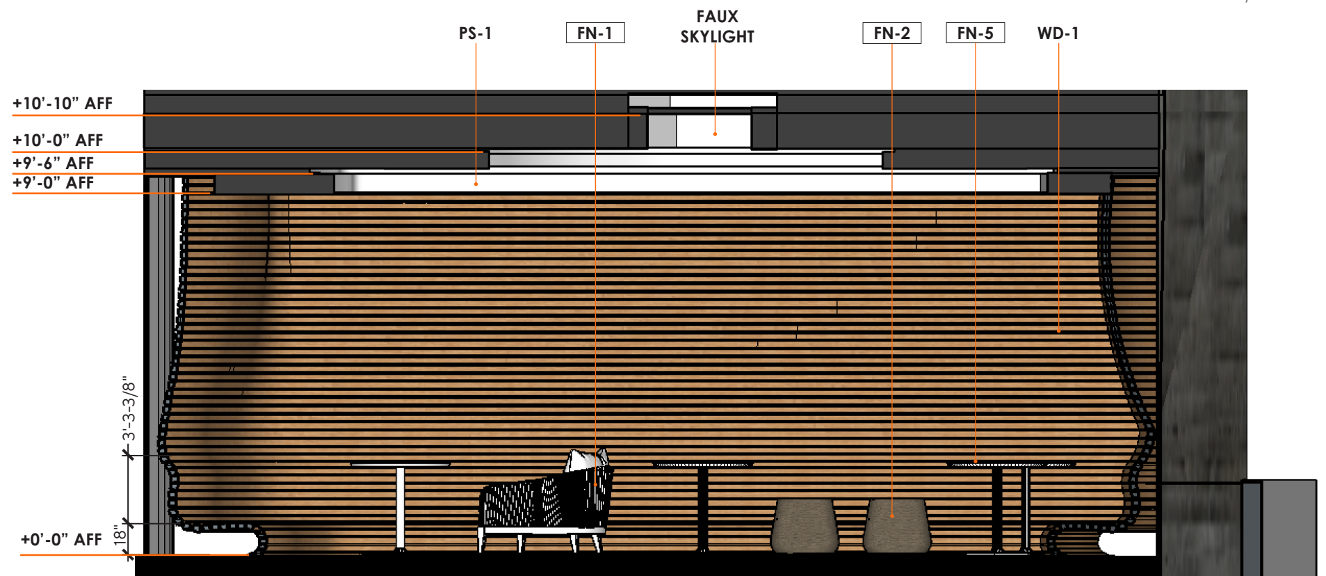
SECTION A2 SCALE: 1/4"=1'-0"
